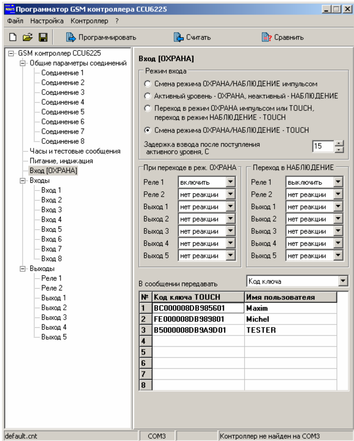
Рисунок 8. Настройка параметров входа "ОХРАНА"
